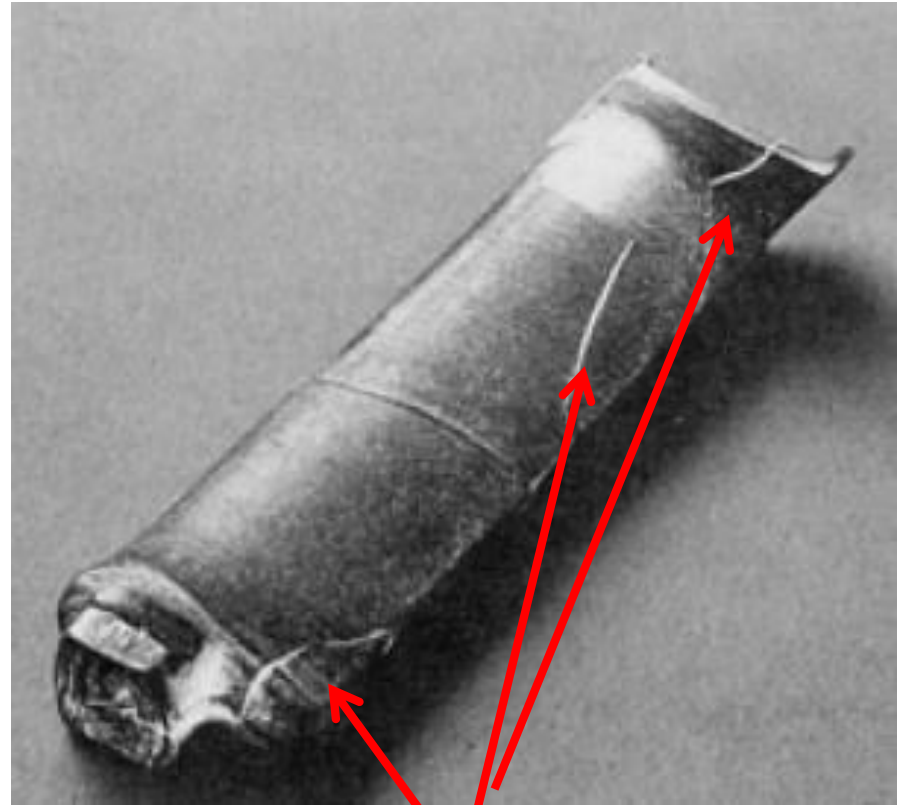
Mikropukotine kompresora otkrivene magnetnim česticama
