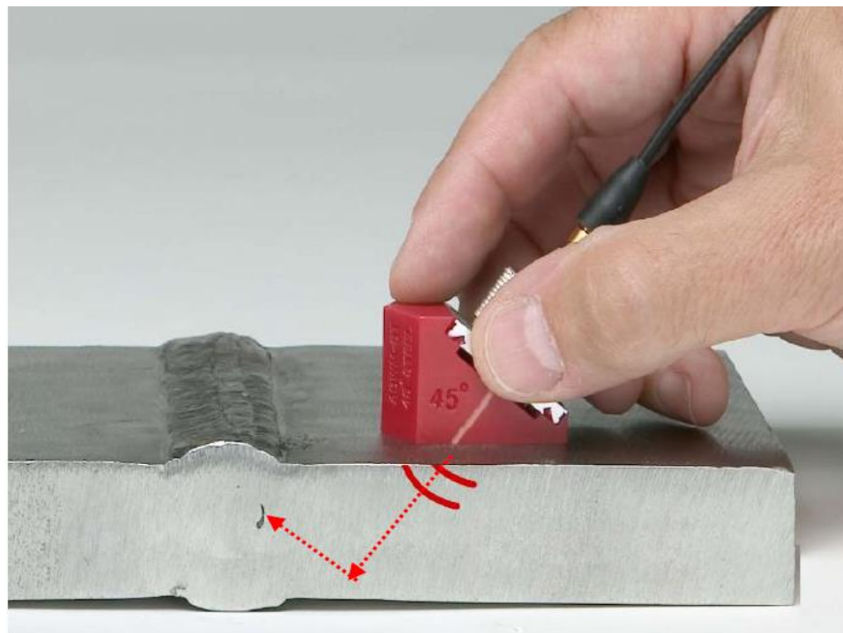
Ultrazvučno ispitivanje zavarenog spoja
